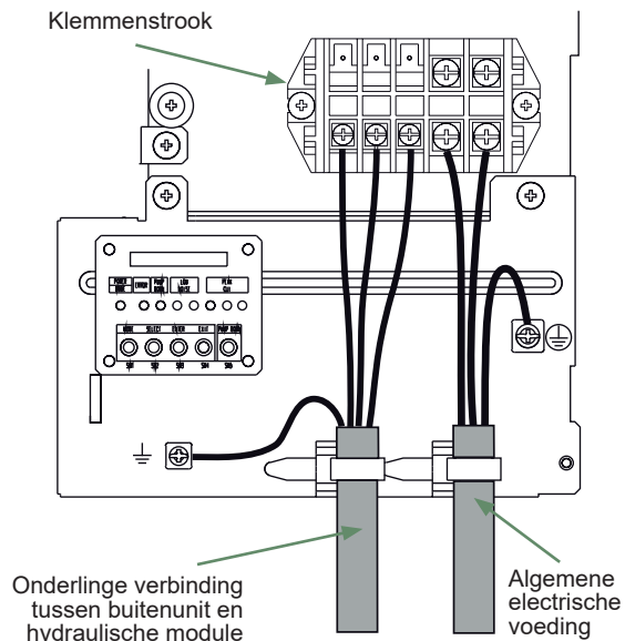
fig. 35 - Aansluitingen op de klemmenstrook van de éénfasige buitenunit
