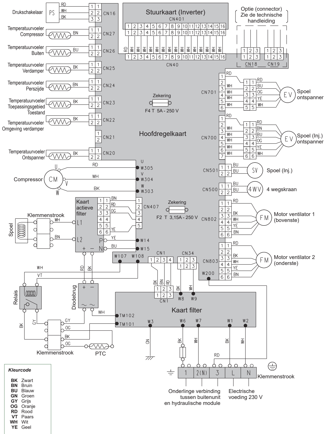
fig. 51 - Elektrisch kablering buitenunit model Alféa Excellia A.I. éénfasig
