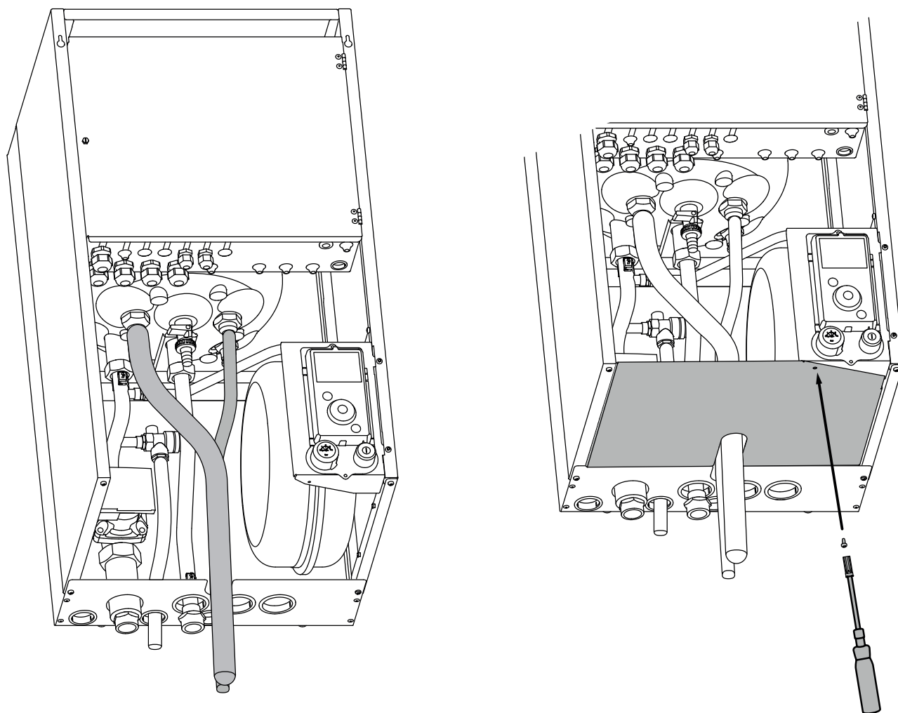
fig. 18 - Doorvoering van de flareverbindingen
