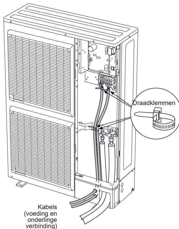
fig. 43 - Voltooiing van de verbinding van de driefasige buitenunit
