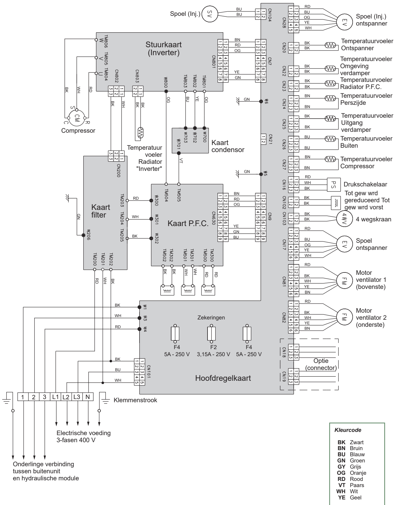
fig. 56 - Elektrische kablering buitenunit model Alfa Excelsia Duo A.I. Driefasig
