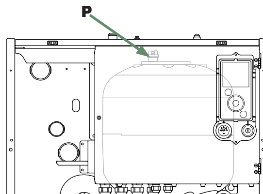
fig. 4 - Automatische ontluchter
