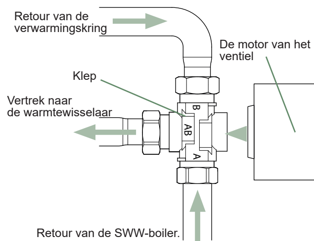
fig. 54 - Montage van de richtingskraan
