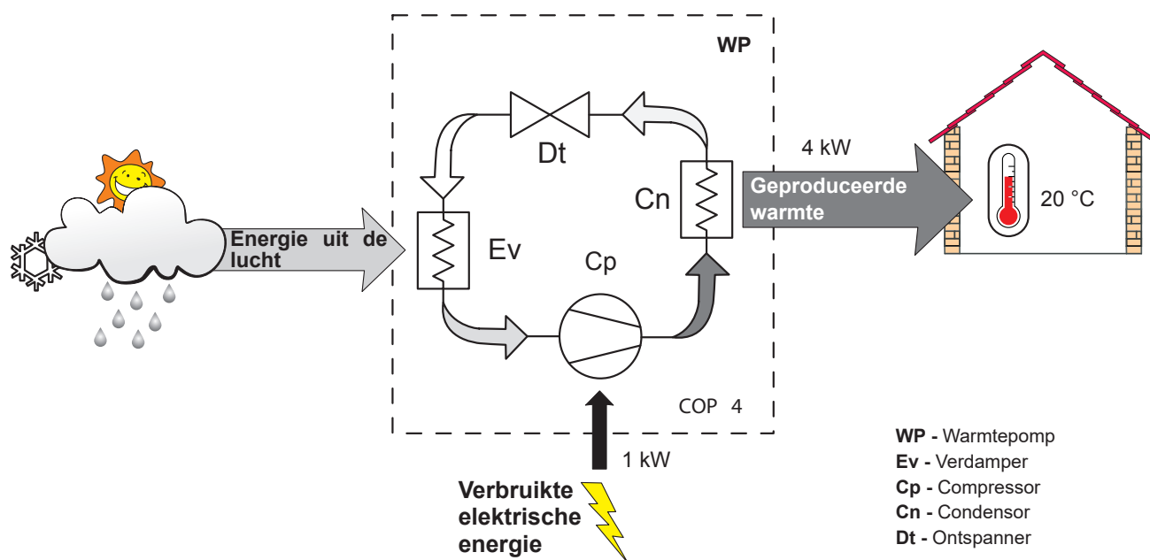
fig. 11 - Weringsprincipe van een warmtepomp
