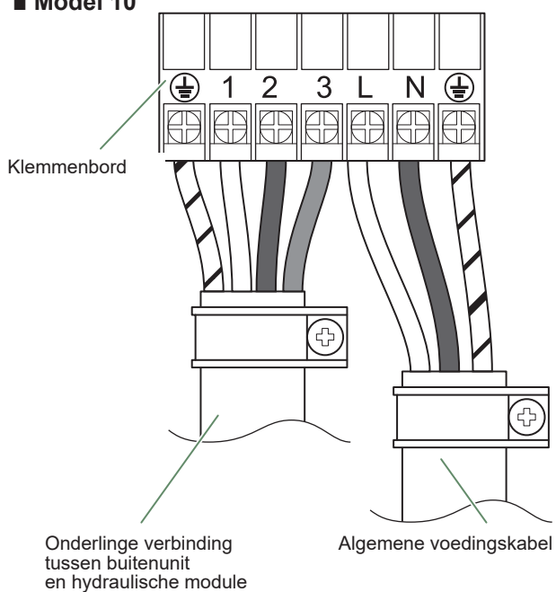
fig. 39 - Aansluitingen op de klemmenstrook van de buitenunit
