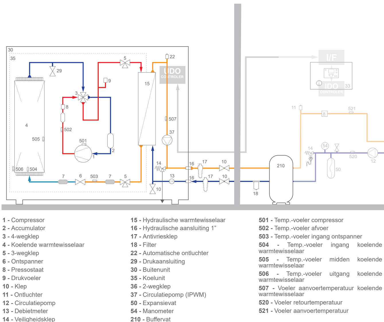
fig. 10 - Hydraulisch prinsipschema
