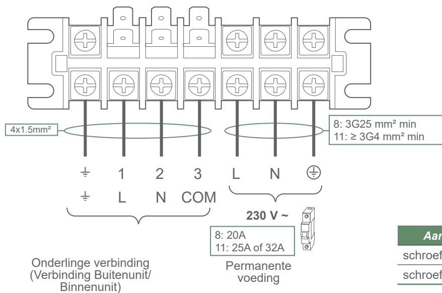
fig. 11 - Klemmenbord elektrische aansluiting zijde buitenunit
