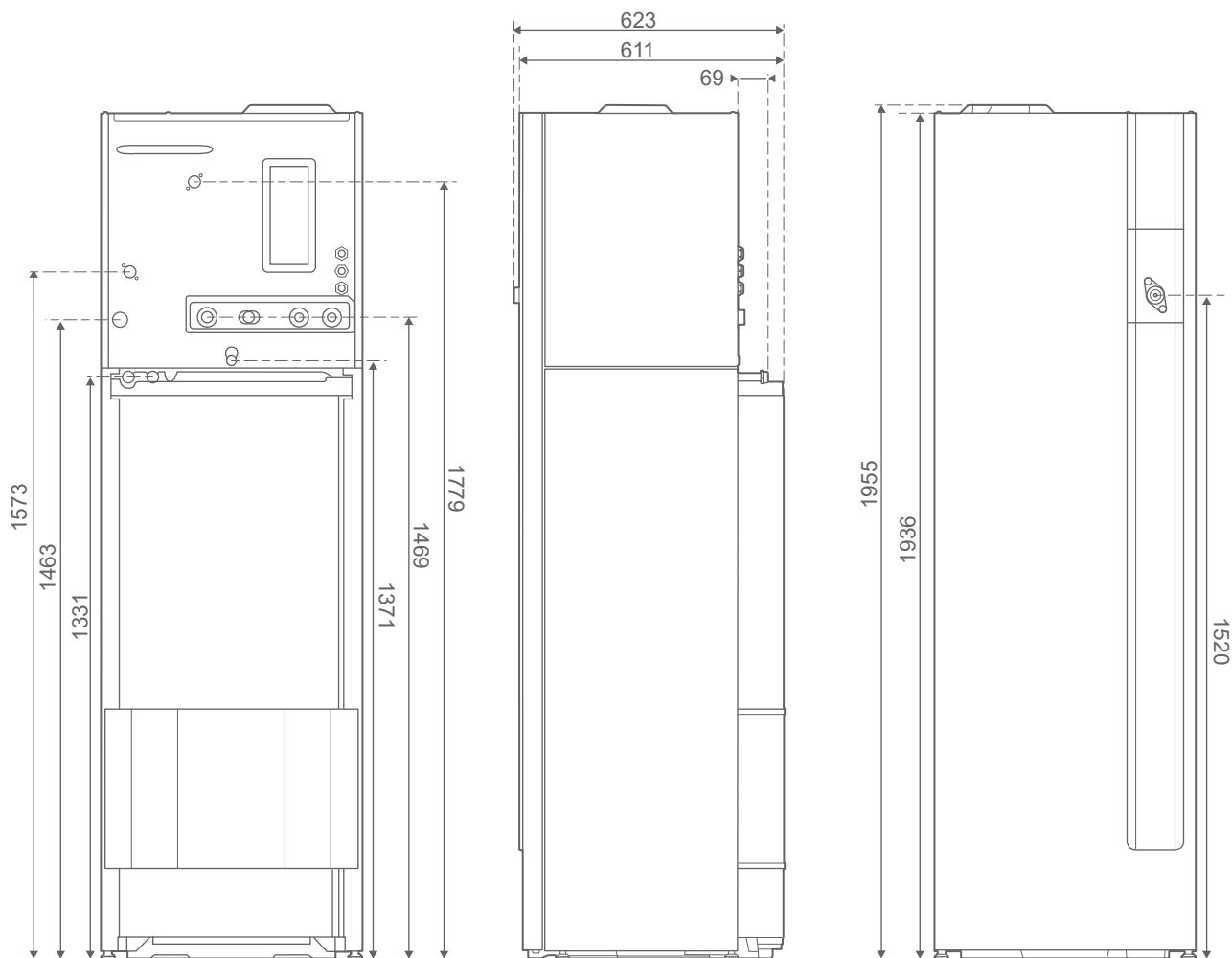
fig. 3 - Afmetingen in mm
