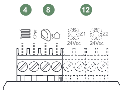
fig. 17 - Aansluitingen Voelers
