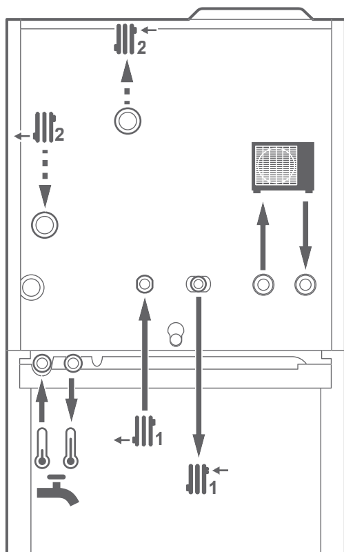
fig. 4 - Hydraulische aansluitingen
