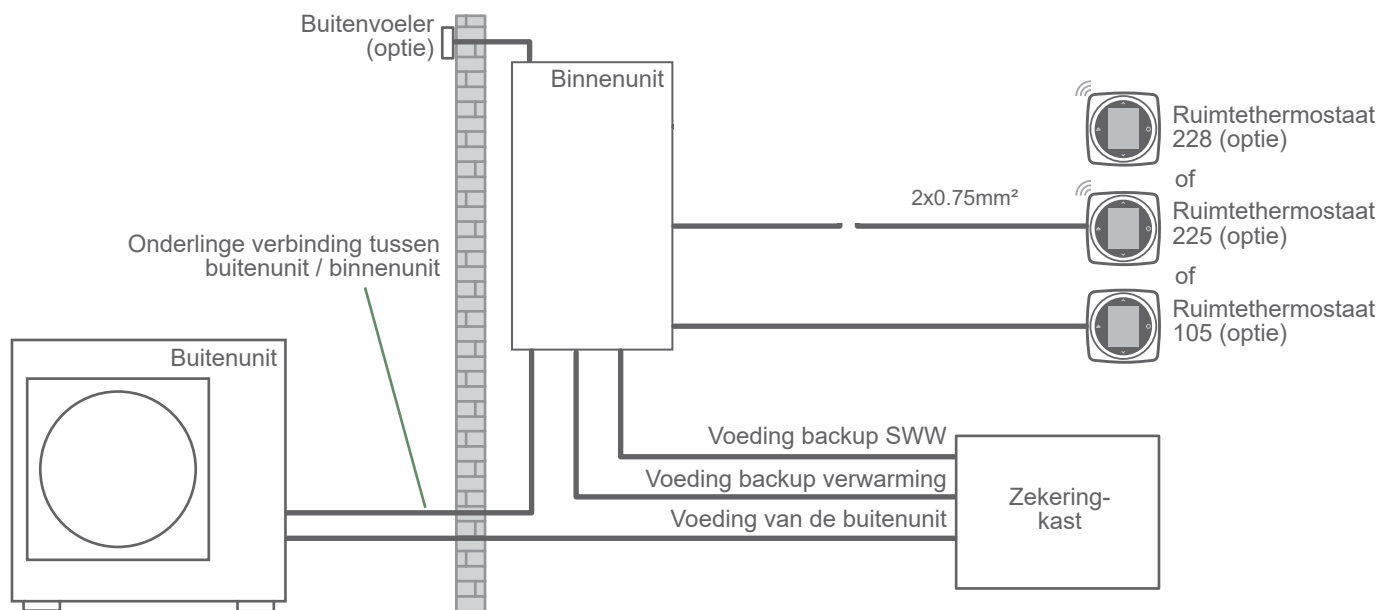
fig. 12 - Overzichtsschema van de elektrische aansluitingen voor een enkelvoudige installatie (1 verwarmingscircuit)
