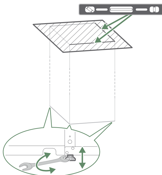
fig. 8 - Waterpas zetten
