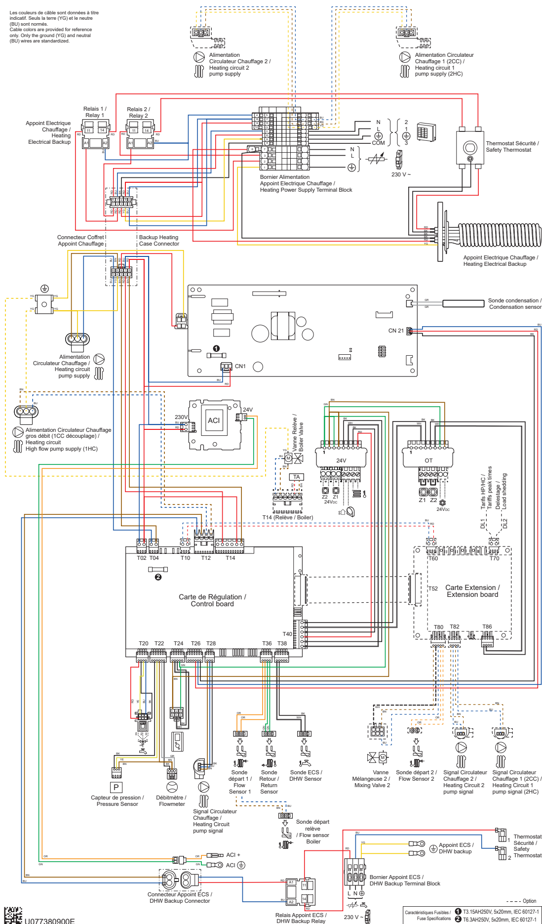
fig. 46 - Elektrische kablering hydraulische module - eenfasig model
