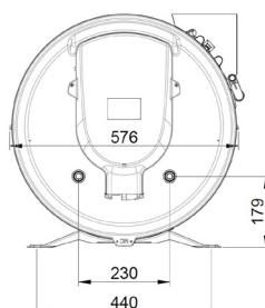
Onderaanzicht
