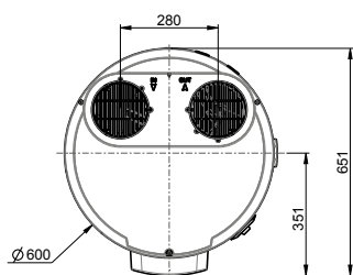
Bovenaanzicht
