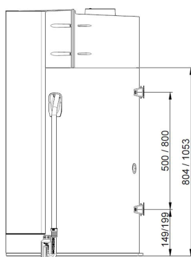
Zijaanzicht rechts
