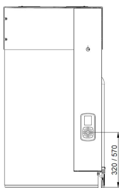
Vooraanzicht
