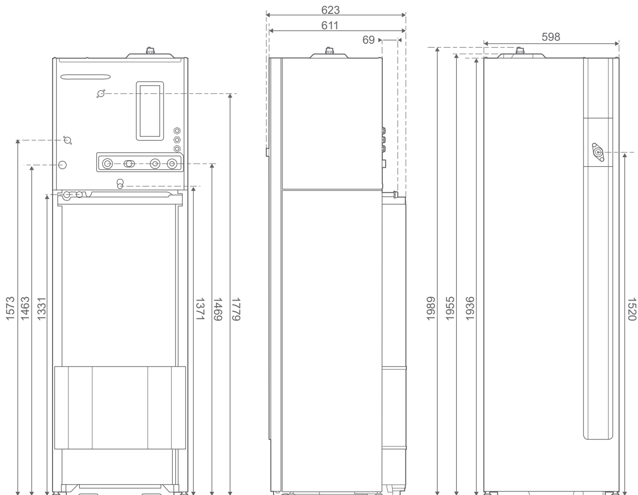
fig. 3 - Afmetingen in mm
