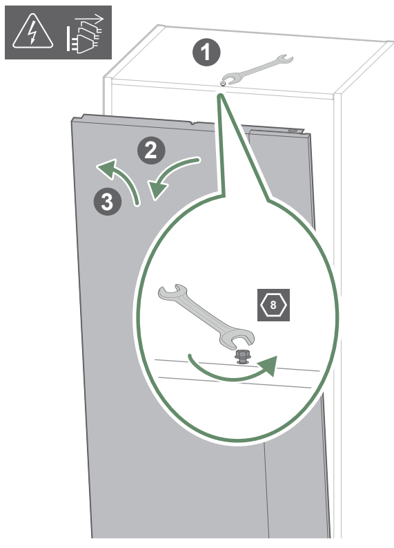
fig. 7 - Opening van het voorpaneel
