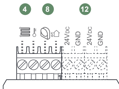
fig. 17 - Aansluitingen sensoren
