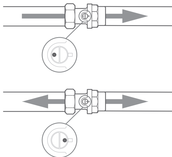
fig. 12 - Terugslagklep
