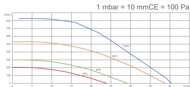
fig. 2 - Hydraulische drukken en debieten beschikbaar
