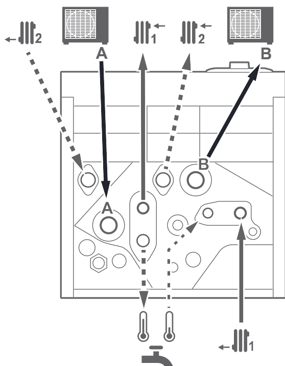
fig. 5 - Hydraulische aansluitingen
