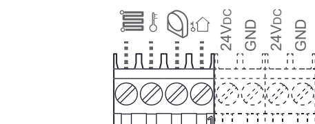
fig. 17 - Voeleraansluitingen
