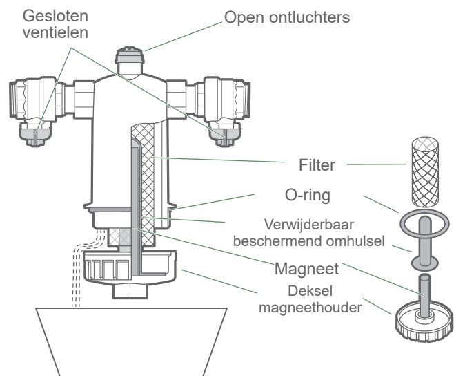
fig. 19 - Vuilfilter reinigen
