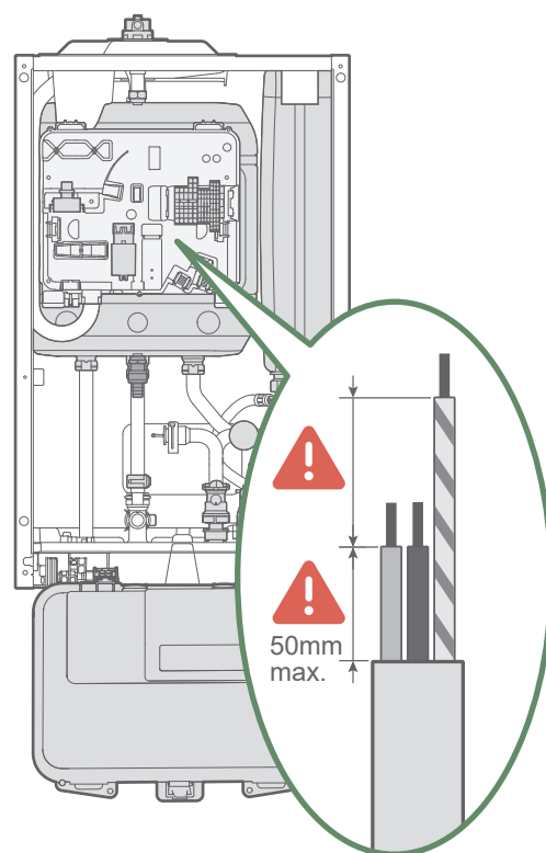
fig. 16 - Kabelgeleiding
