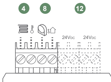
fig. 42 - Voeleraansluitingen
