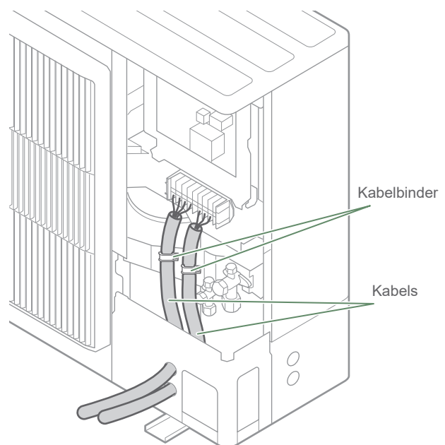
fig. 40 - Toegang tot aansluitingsklemmen van de buitenunit
