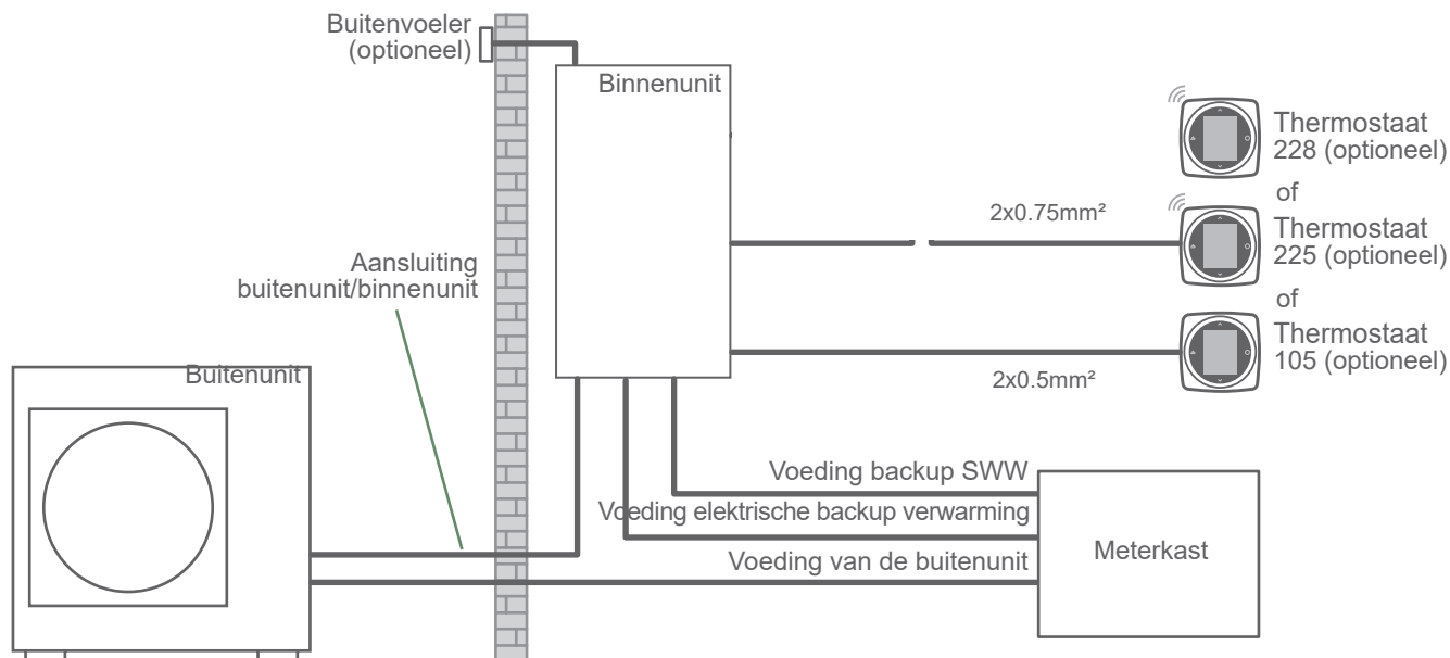
fig. 37 - Overzicht van elektrische aansluitingen voor eenvoudige Installatieruimte (1 verwarmingscircuit)
