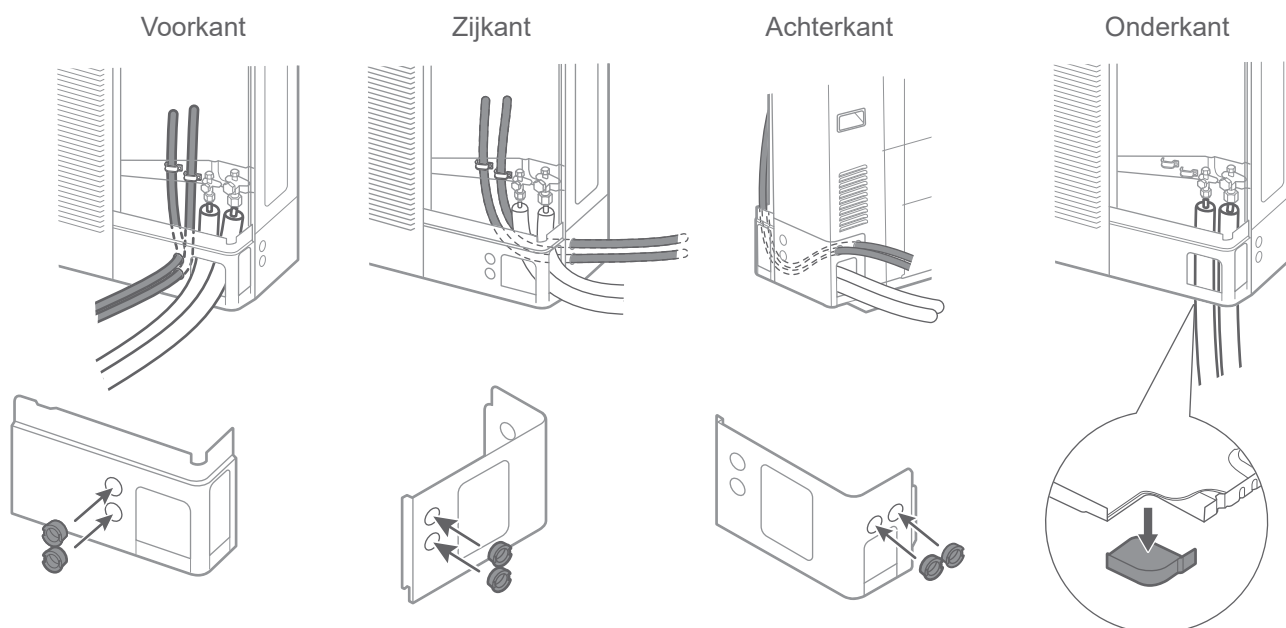
fig. 30 - Doorgang van de koelaansluiting van de buitenunit.
