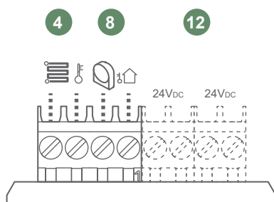
fig. 40 - Voeleraansluitingen
