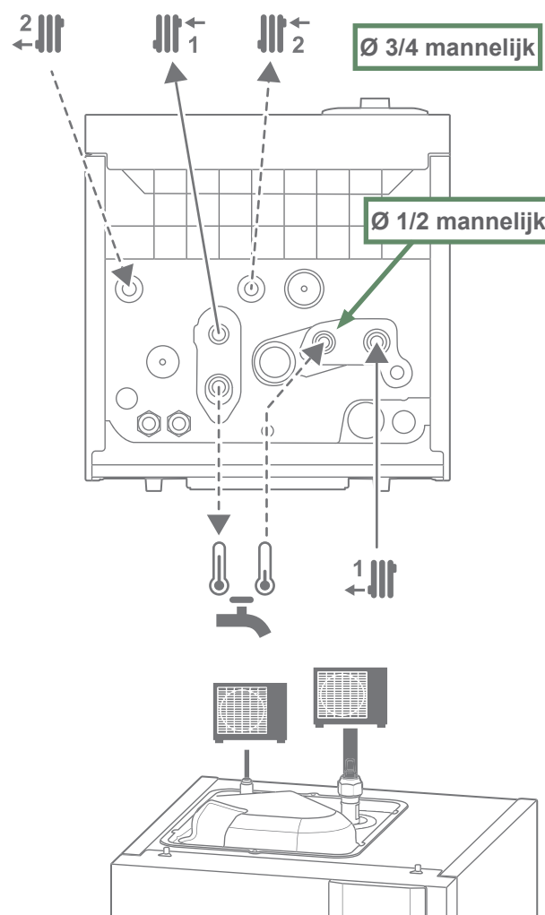
fig. 2 - Hydraulische marking
