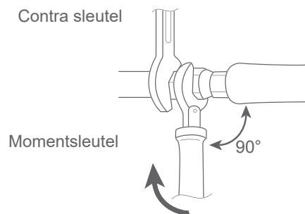
fig. 29 - Aanhaalmoment
