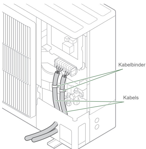
fig. 38 - Toegang tot aansluitingsklemmen van de buitenunit
