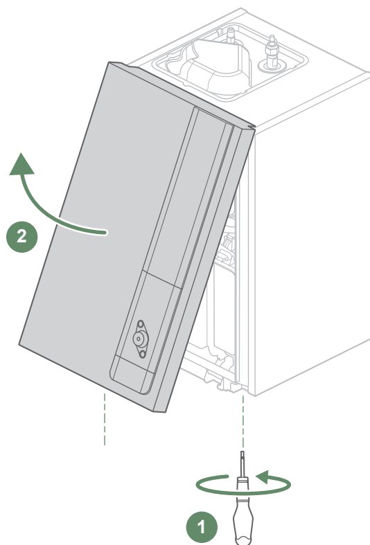
fig. 19 - Opening van het voorpaneel
