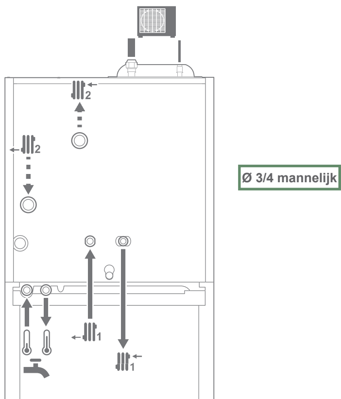
fig. 3 - Hydraulische aansluitingen
