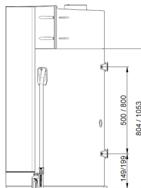
Zijaanzicht rechts
