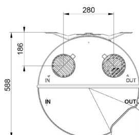
Bovenaanzicht
