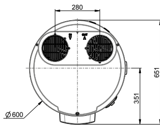
Bovenaanzicht
