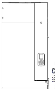
Vooraanzicht
