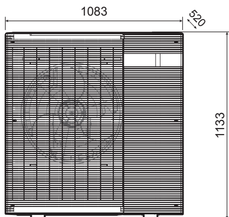
Buitenunit - vooraanzicht
